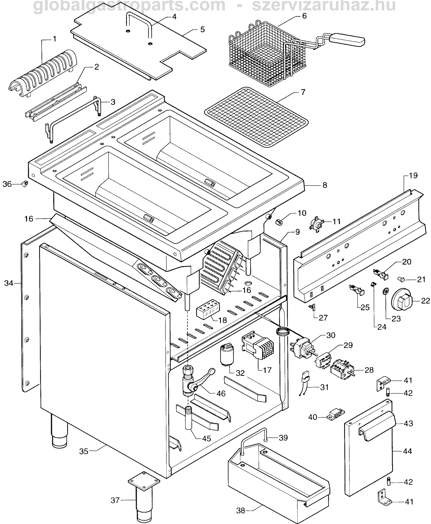
FRIGGITRICE ELETTRICA 8 L PR 700 ELETTRICA FRYER 8 L
