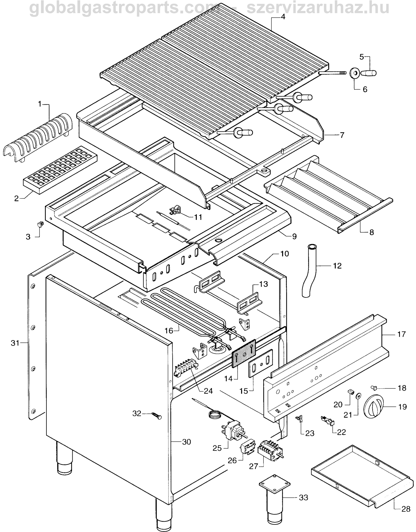
GRIGLIA ELETTRICA ELECTRIC GRILL PR 700
